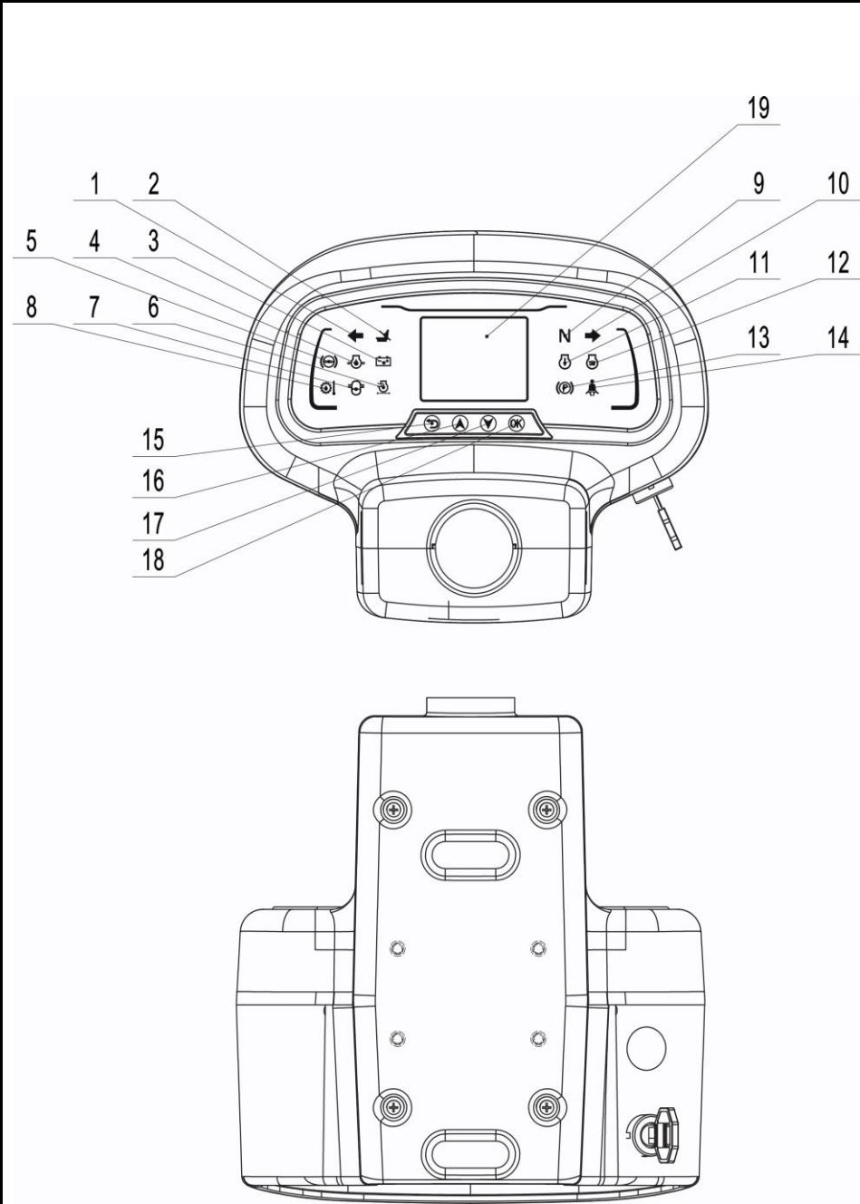
图13-D 仪表总成 Figure13-D Meter assembly 293333510021
